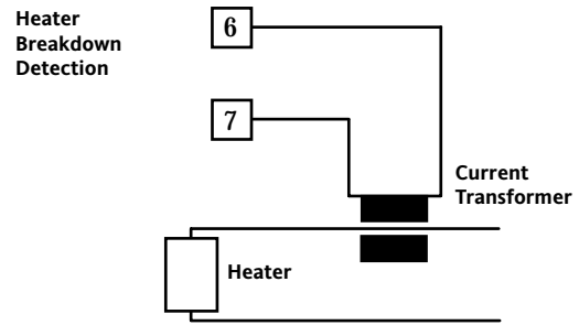
CT Part Number: 7ER-Rx000-000 x = 1 (10A); x = 2 (25A); x = 4 (50A); x = 5 (100A)
